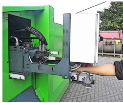
El- og hydraulikaggregat på udtrækkelig skinne for lettere service
